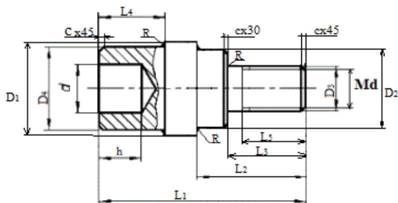
Рис.13 – Эскиз детали
