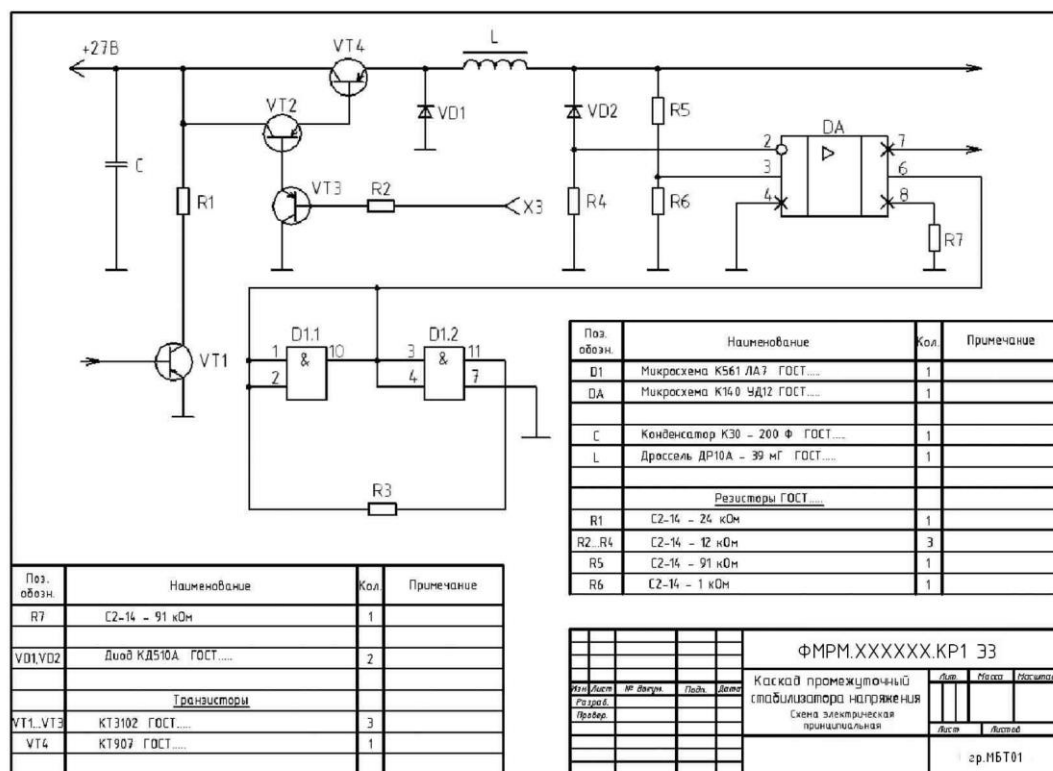
Электрическая принципиальная схема
